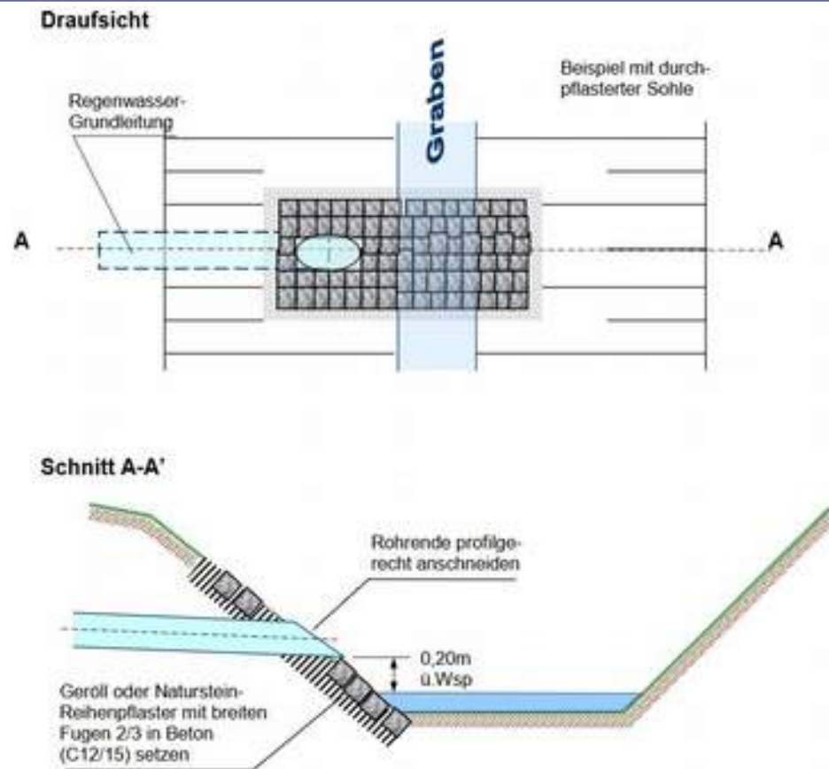
Prinzipskizze
